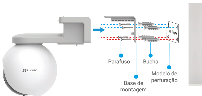
Fig. 2 Montagem na parede
